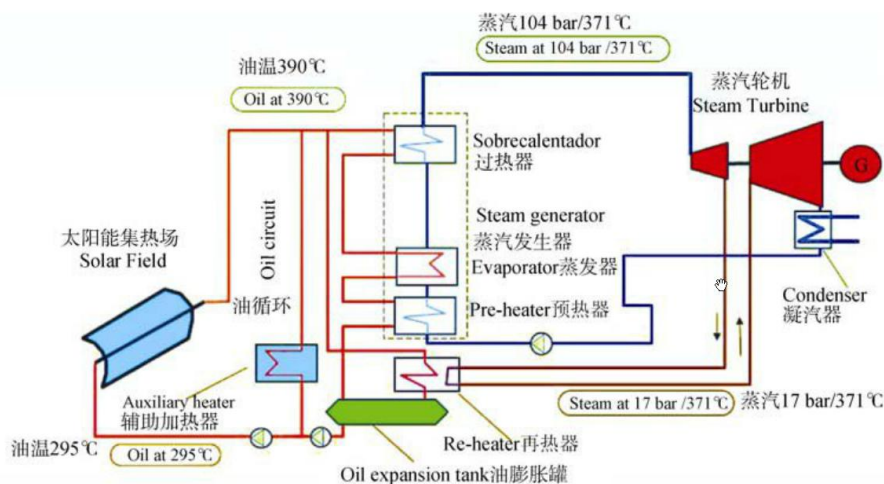
图1 槽式太阳能电站示意图 [3]
